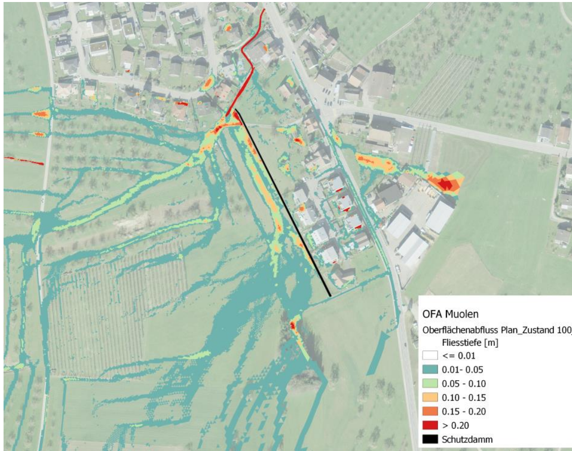
Abbildung: Fliesstiefen Plan-Zustand mit Schutzdamm
