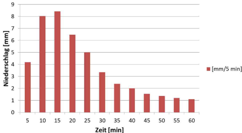
Abbildung: Ganglinie 100-jährliches Ereignis [1]
