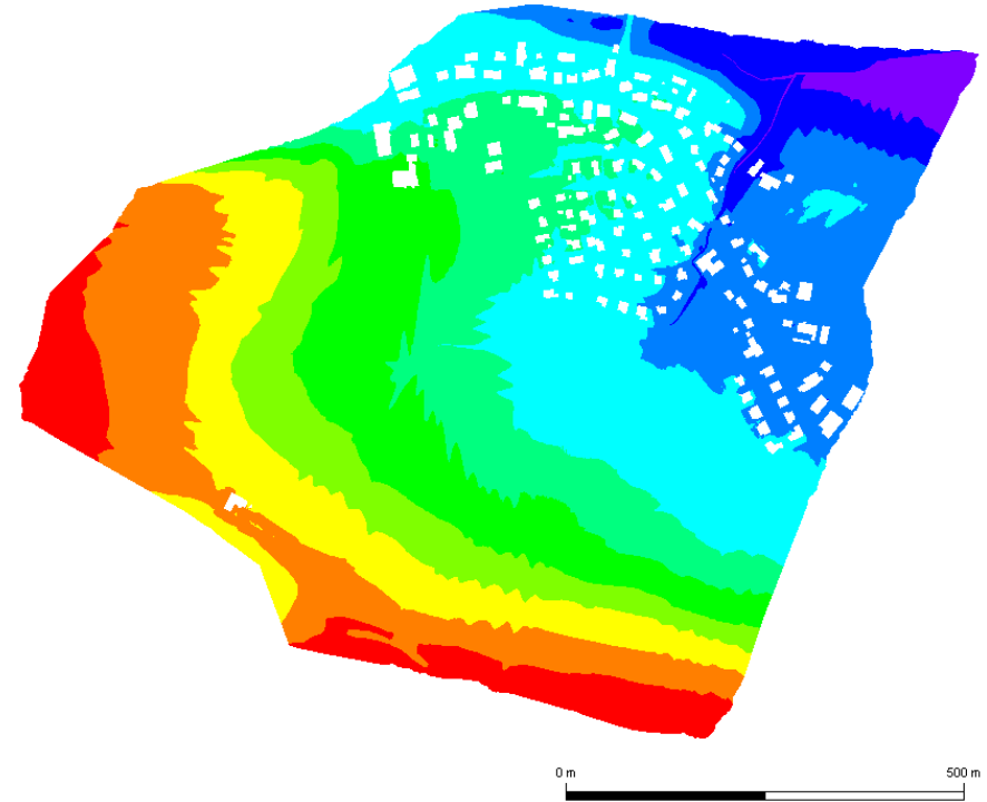
Abbildung: 2D-Oberflächenabflussmodell
