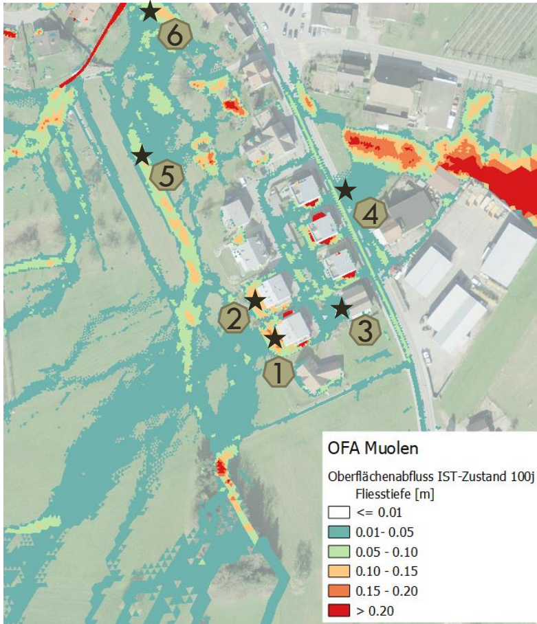
Abbildung: Fliesstiefen IST-Zustand
