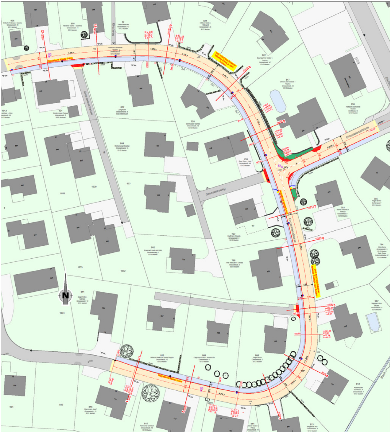
Plan Strassen- und Werkleitungssanierung Grosswiesstrasse, unmassstäblich
